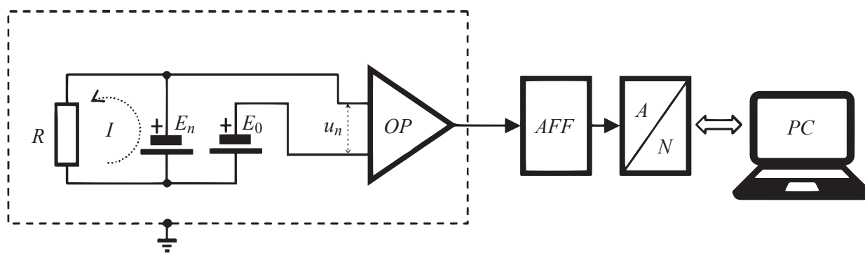
Рис. 1. Функциональная схема установки для флуктуационно-шумовых измерений: E_n и E_0 – исследуемый и компенсирующий элементы ХИТ; u_n – регистрируемый флуктуационно-шумовой сигнал; R и I – нагрузочное сопротивление и ток разряда; OP , AAF , A/N и PC – усилитель, фильтр, аналого-цифровой преобразователь и компьютер в измерительном тракте
