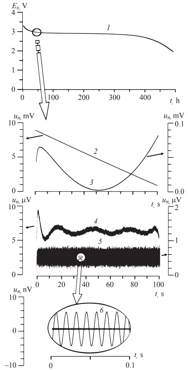
Рис. 2. Флуктуационно-шумовой сигнал на различных этапах предобработки: 1 – общая разрядная кривая E(t) и её фрагмент (выделен кружком); 2, 3, 4 и 5 – флуктуационно-шумовой сигнал u(t) соответственно в исходном виде, после линейного фитинга, после полиномиального и сплайнового фитинга; 6 – тестовый сигнал малой амплитуды после его фильтрации
